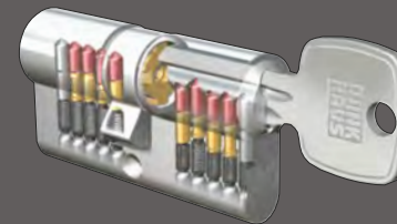
K 20 / Not- und Gefahrenfunktion mit 6 Schlüsseln
